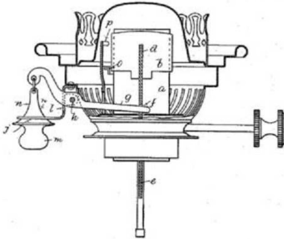
Hins & Sons , seccion transversal, movimiento 1 del apaga llamas, abierto
